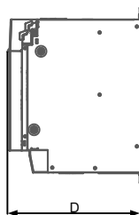
Рис. 1-4 Габаритные размеры модуля инвертора (двухосевой)
