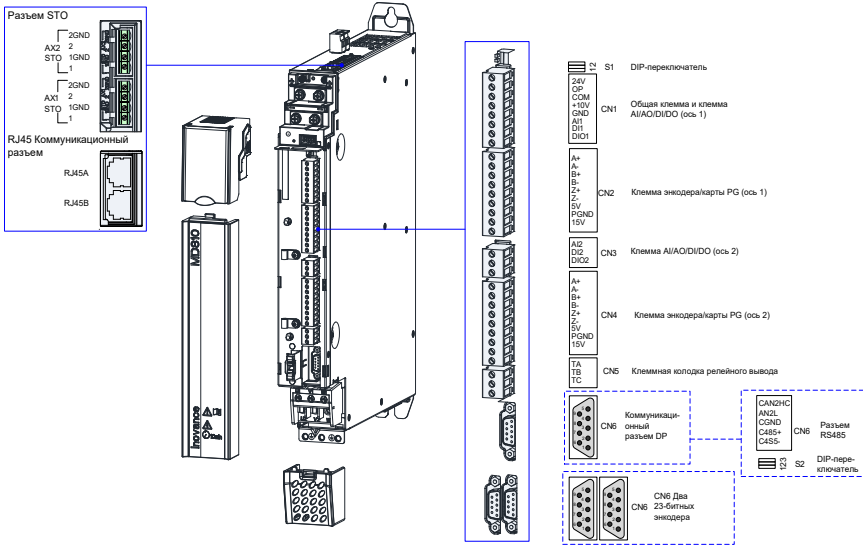
Рис. 3-5 Расположение клемм цепи управления модуля инвертора (двухосевой)
