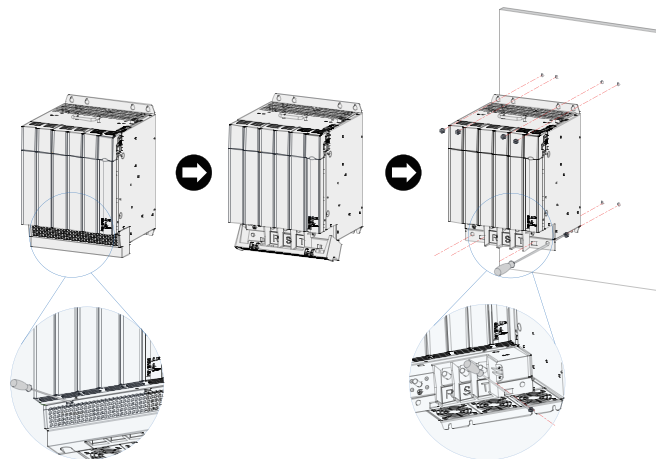
Рис. 2-4 Установка на монтажную панель MD810-50M4T90G–MD810-50M4T160G
