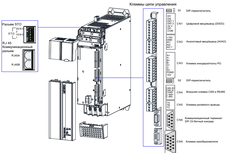
Рис. 3-3 Расположение клемм цепи управления модуля инвертора (одноосевой, книжный формат, 1,5 – 160 кВт)
