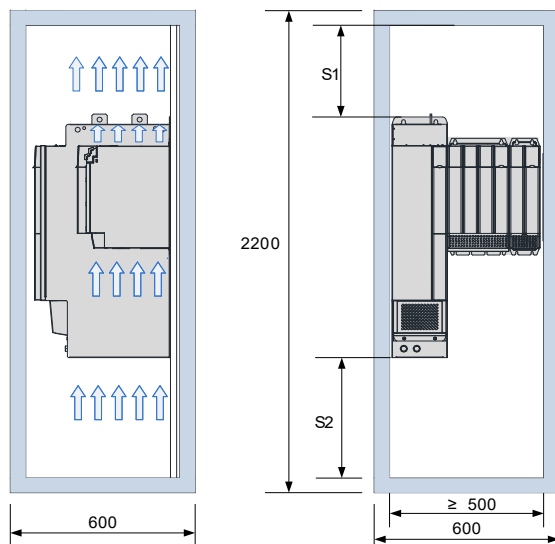
Рис. 2-2 Свободное пространство для рассеивания теплоты для модуля источника питания высокой мощности (вертикальный блок)
