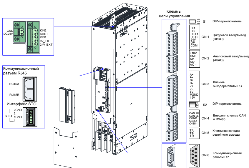
Рис. 3-4 Расположение клемм цепи управления модуля инвертора (одноосевой, книжный формат, 90–355 кВт, вертикальное исполнение)
