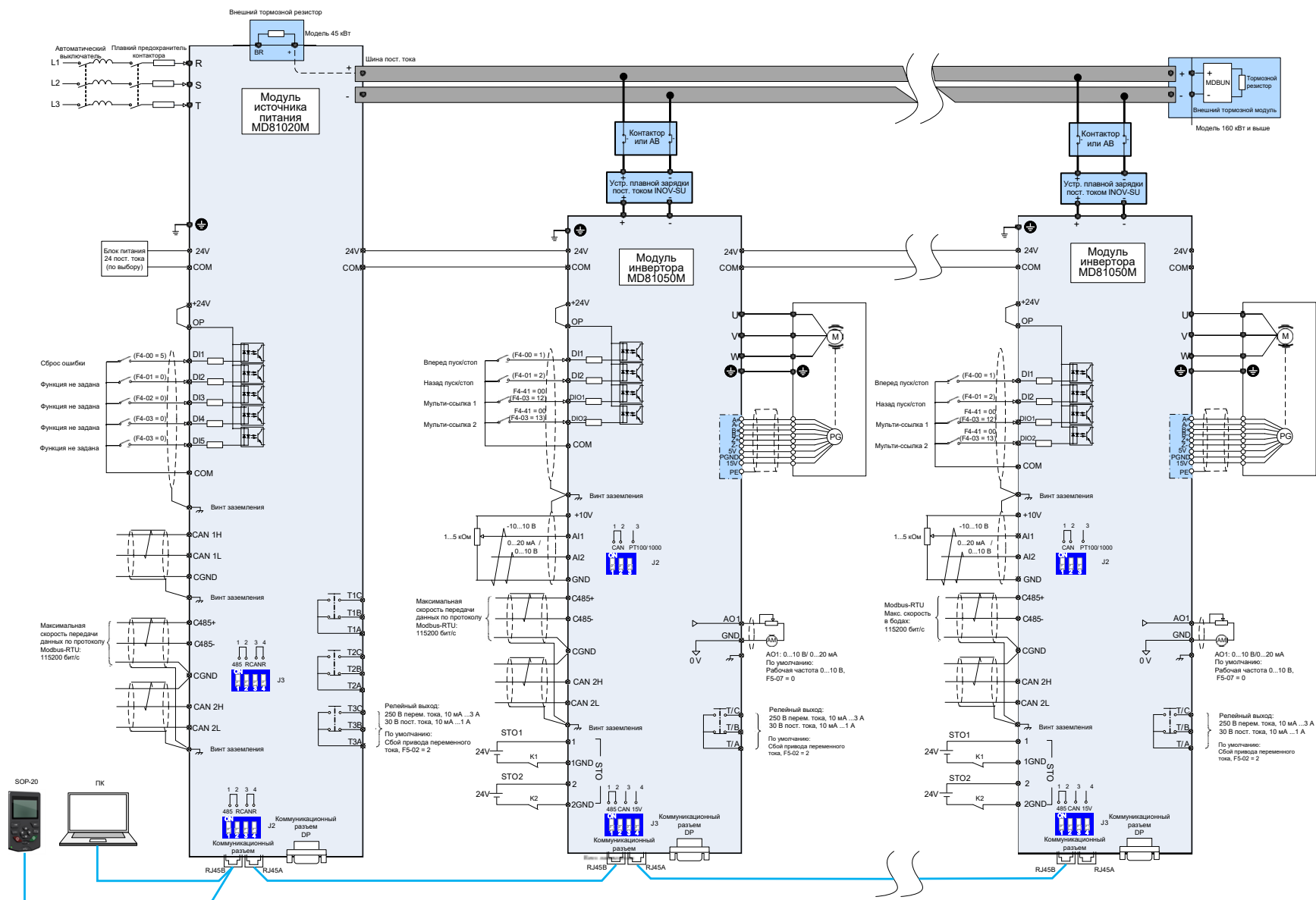
Рис. 3-6 Электромонтажная схема типовой системы
