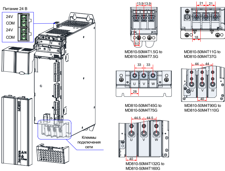
Рис. 3-1 Расположение клемм питания и размер модуля инвертора (одноосевой)
