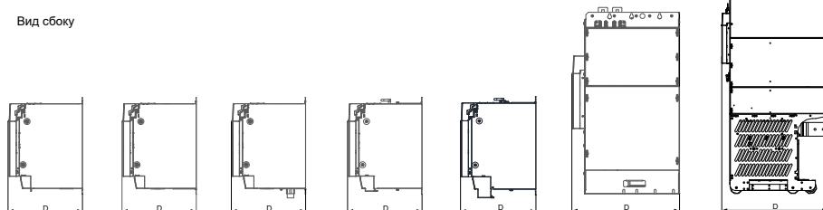
Рис. 1-3 Габаритные размеры модуля инвертора (одноосевой)
