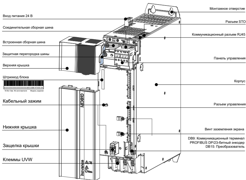
Рис. 1-2 Узлы и детали модуля инвертора
