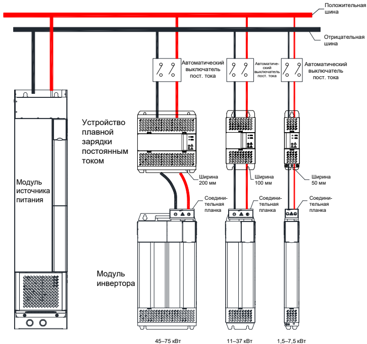
Рис. 2-6 Монтаж устройства плавной зарядки постоянным током INOV-SU-30/INOV-SU-60/INOV-SU-100/INOV-SU-170
