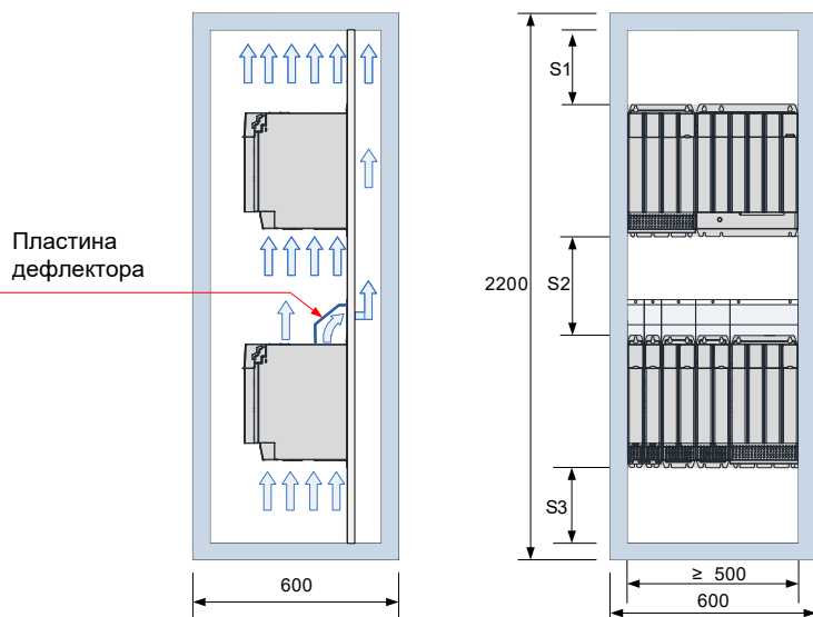
Рис. 2-1 Свободное пространство для модулей книжного формата при монтаже в две стойки
