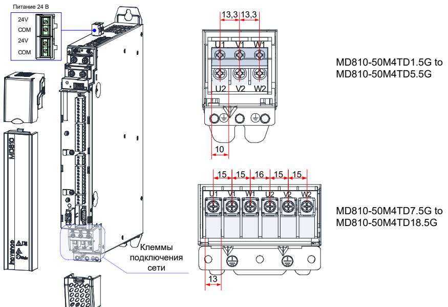
Рис. 3-2 Расположение клемм питания и размер модуля инвертора (двухосевой)
