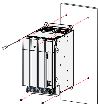
Рис. 2-3 Установка на монтажную панель MD810-50M4T45G–MD810-50M4T75G
