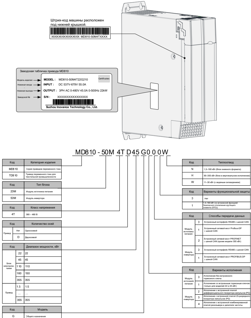
Рис. 1-1 Заводская табличка и код модуля инвертора
