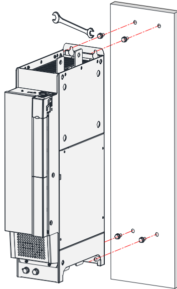
Рис. 2-5 установка на монтажную панель MD810-50M4T90G–MD810-50M4T160G
